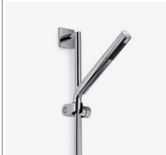
26 402 780 Complete shower set Gruppo doccia con flessibile e asta saliscendi Juego de ducha de mano con barra corredera [14 l/min.]
