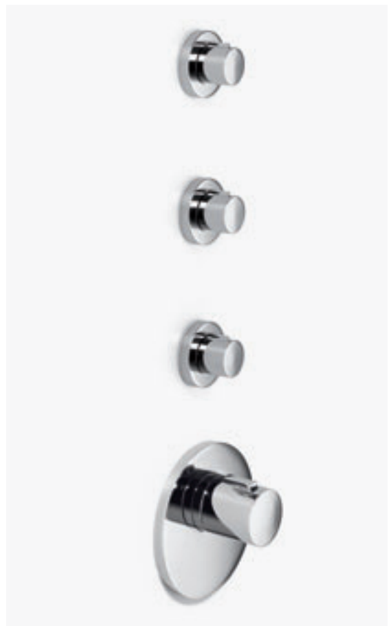
36 416 979* + 3x 36 310 979* / + 2x 36 310 979* / + 1x 36 310 979* xTool thermostat module with 3 valves/2 valves/1 valve xTool modulo termostato con 3 rubinetti/2 rubinetti/1 rubinetto Módulo de termostato xTool con 3 válvulas/2 válvulas/1 válvula
