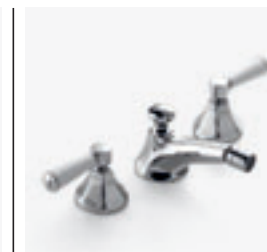
13 900 380 + 20 000 370 + 2x 04 23 30 040 00 00 + 2x 12 501 970 90 Three-hole bidet mixer Batteria tre fori bidet Bateria americana de bidet [7 l/min.]
