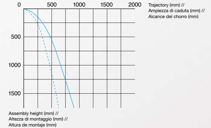
Trajectory // Ampiezza di caduta // Alcance del chorro
