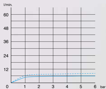
Flow rate // Flusso // Caudal
